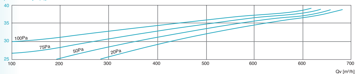
Lp1m intérieur [dB(A)]
